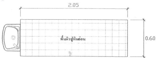
แบบขยายเคาน์เตอร์ 2 มาตราส่วน 1 : 25
