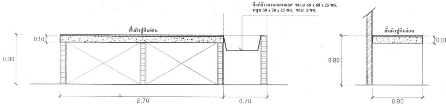
รูปตัดขยายเคาน์เตอร์ 1 มาตราส่วน 1 : 25
