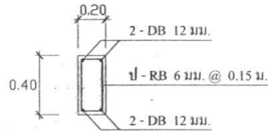
B1 มาตราส่วน 1 : 25
