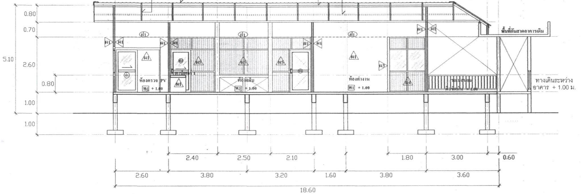
รูปตัด (B-B) มาตรฐาน 1 : 75
