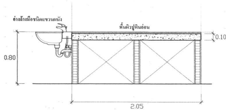
รูปตัดขยายเคาน์เตอร์ 2 มาตราส่วน 1 : 25
