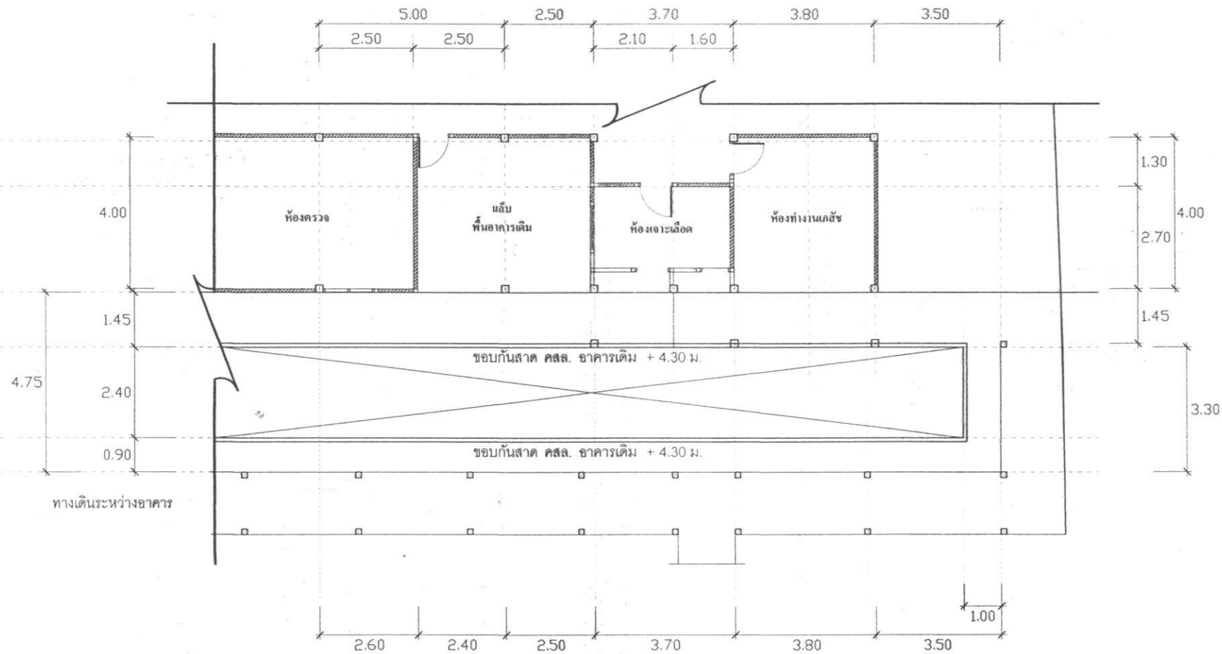
แปลนกันสาดอาคารเดิม มาตรฐาน 1 : 100
