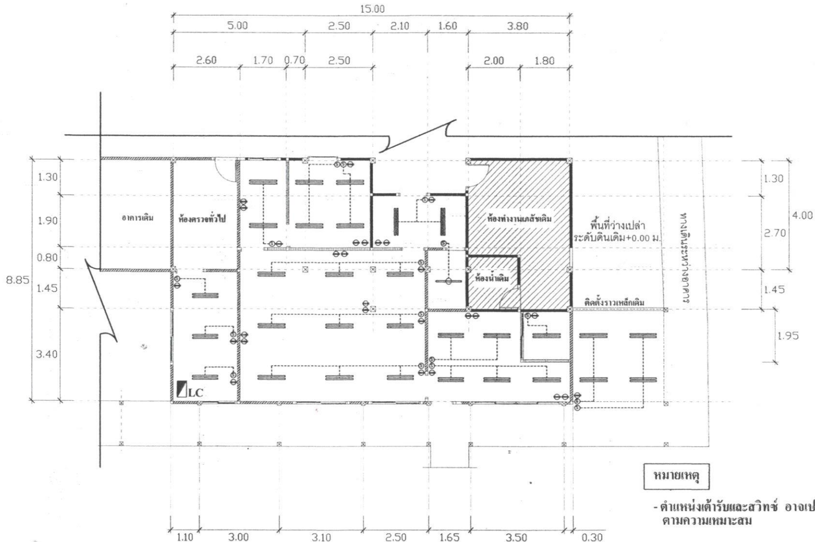
แปลนระบบไฟฟ้า มาตรฐาน 1 : 100
