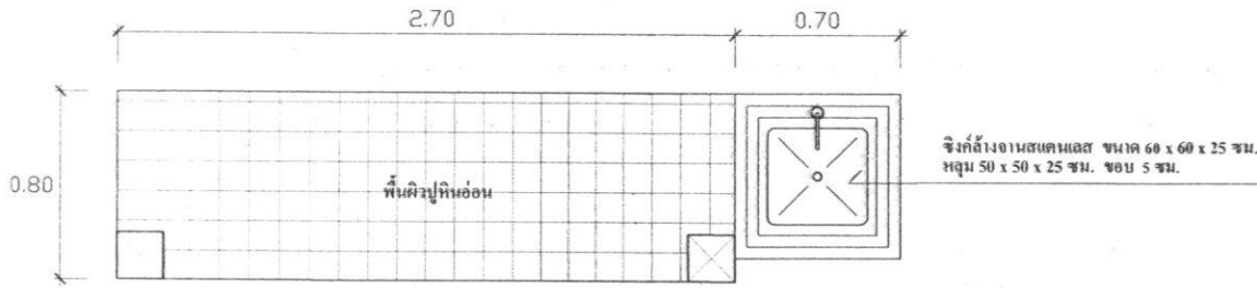
แบบขยายเคาน์เตอร์ 1 มาตราส่วน 1 : 25
