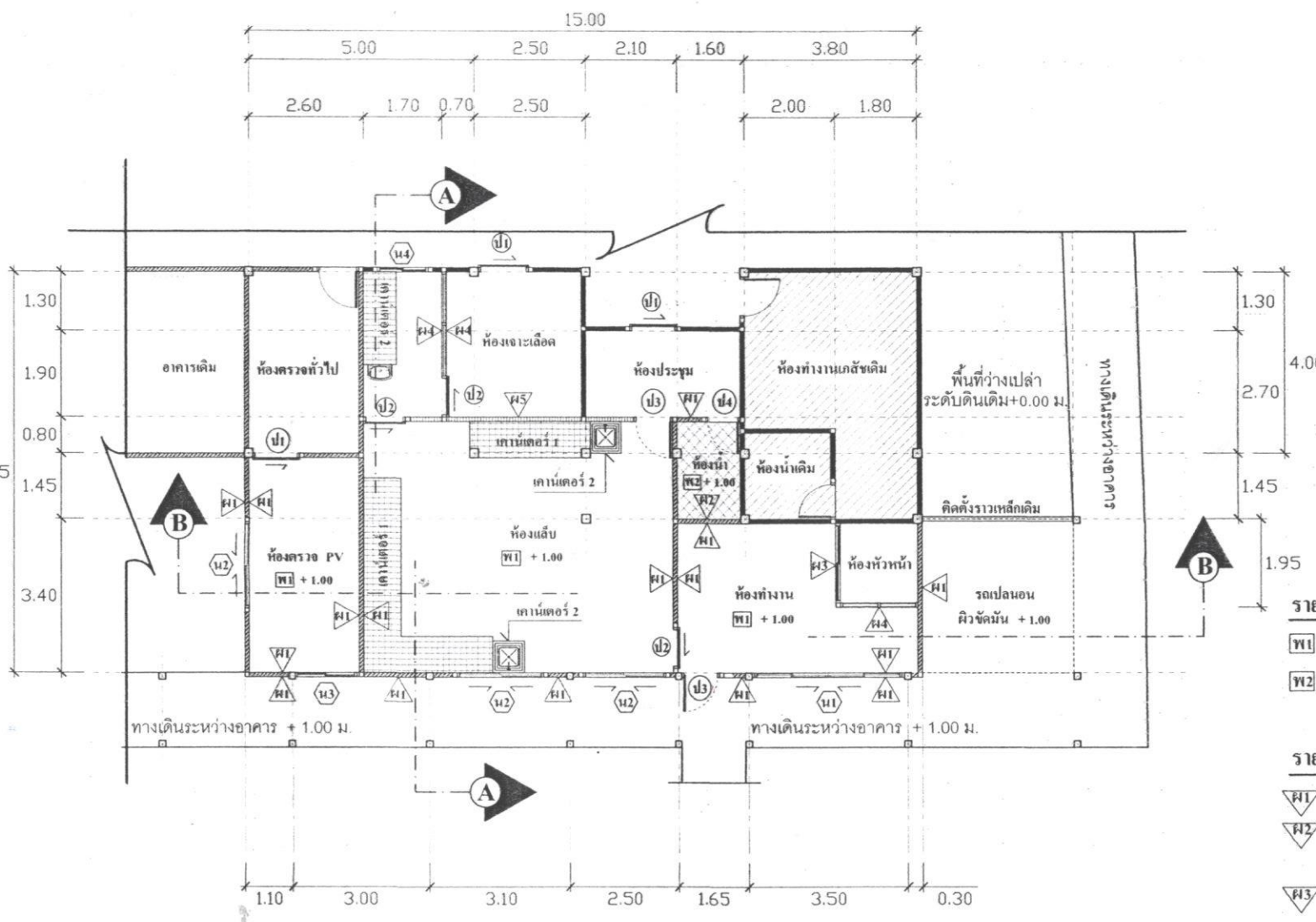
แปลนปรับปรุงอาคาร มาตรฐาน 1 : 100
