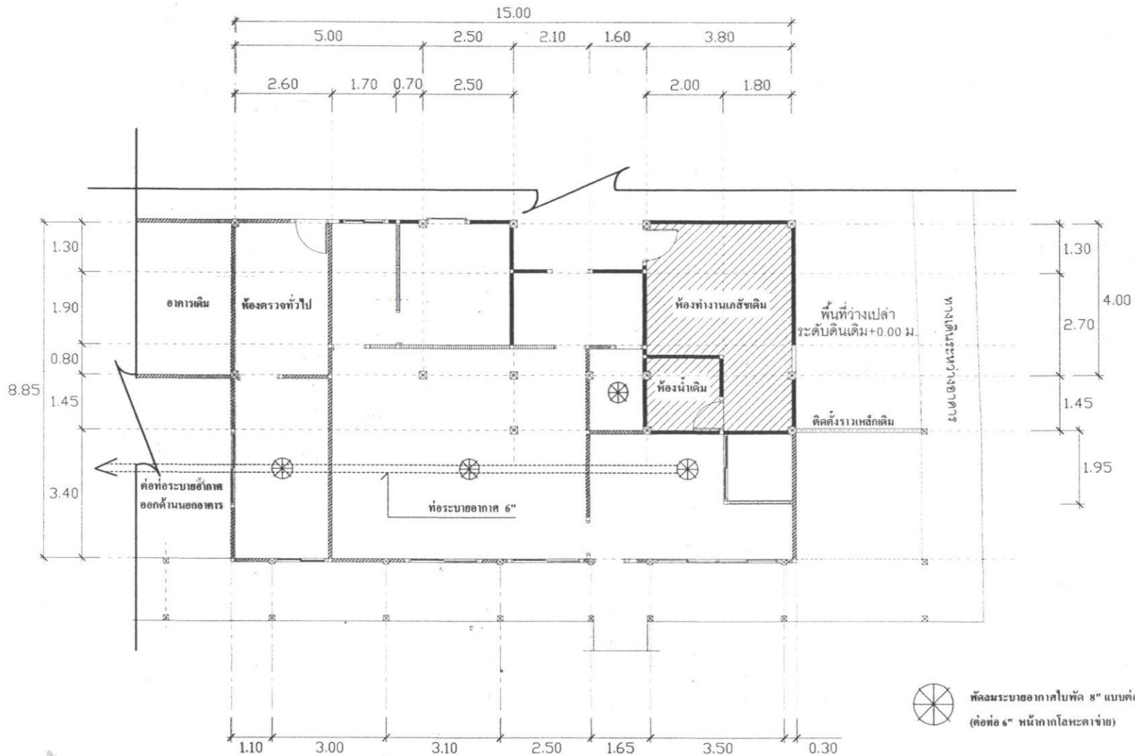
แปลนระบบระบายอากาศ มาตรฐาน 1 : 100
