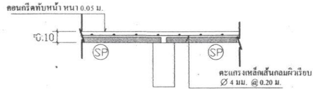
ลักษณะการวางพื้น (SP) มาตราส่วน 1 : 25
