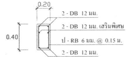
B2 มาตราส่วน 1 : 25
