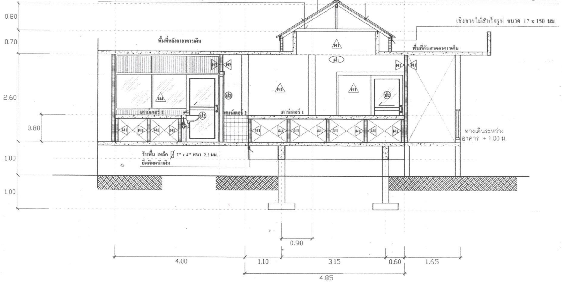
รูปตัด A-A มาตรฐาน 1 : 50
